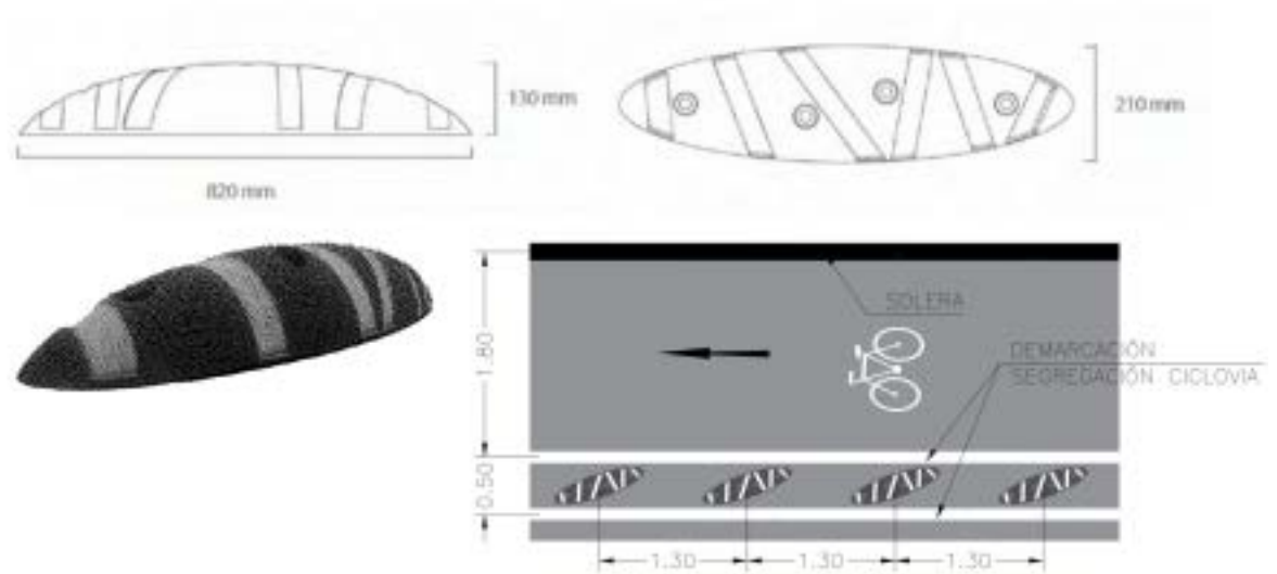
Figura 6-2 Detalle canalizado ciclovía
