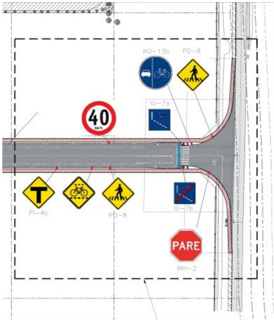
Figura 5-4 Intersección nueva ciclovía proyectada con caldera poniente ruta Los Libertadores
